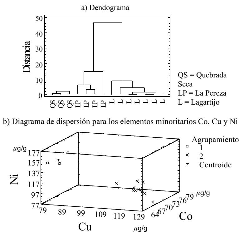
Figura 2. Dendrograma y diagrama de dispersión para los elementos minoritarios.
