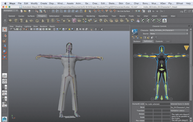
Figura 2. Interface de Autodesk Maya con la pestaña Human IK desplegada. Se puede observar, a la izquierda, el modelo del Avatar con sus huesos. En el recuadro de la derecha se aprecia cómo esos huesos influyen sobre la malla poligonal de acuerdo a parámetros estandarizados de captura de movimiento ( MoCap ).
